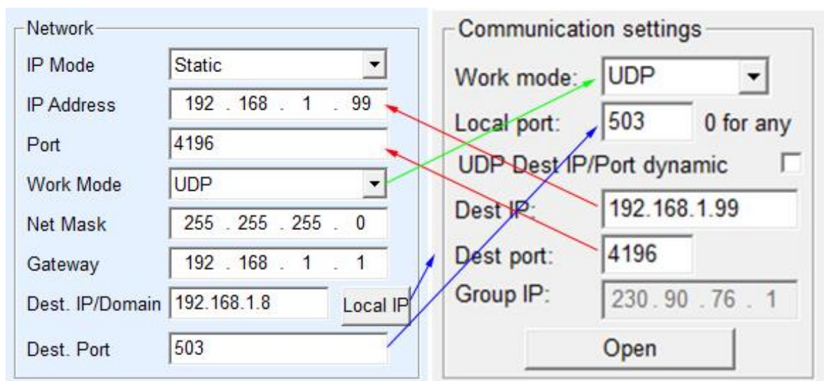
Figure 28 UDP mode Parameter Configuration
